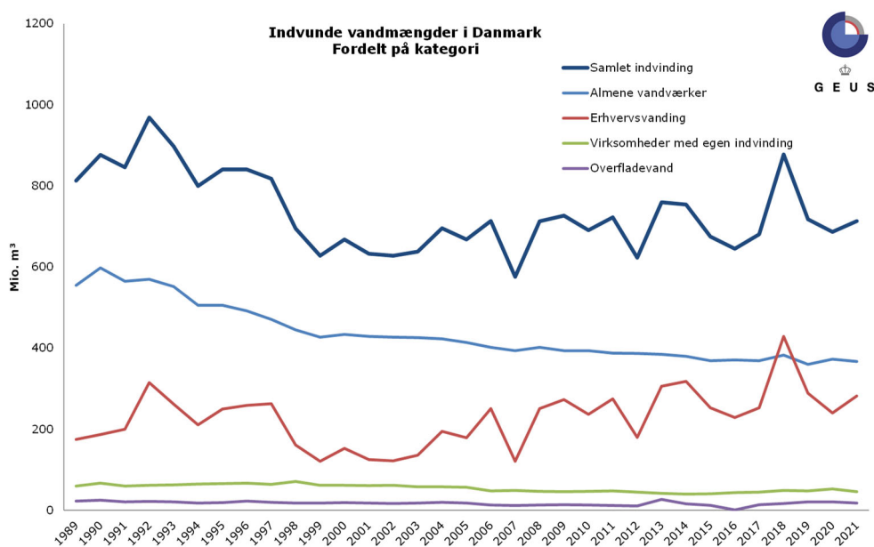
Figur 23. Vandindvinding i Danmark i perioden 1989-2021 opdelt på almene vandværker, erhvervs vand, industri og overfladevand. Den samlede indberettede indvinding er vist med en fed, mørkeblå linje. Bemærk, hvorledes den varierer med erhvervs vand, hvoraf markvanding udgør hovedparten.
