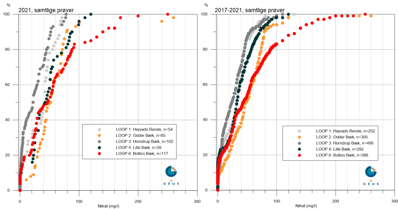
Figur 32. LOOP. Fordelingen af nitratkoncentrationen fra LOOP i samtlige prøver fra 2021 (til venstre) og i perioden 2017-21 (til højre) i de 5 målte LOOP-områder afbildet i et fraktildiagram. Grålige signaturer viser lerjordsområder: LOOP 1, 3 og 4, mens rødlige signaturer viser sandjordsområder: LOOP 2 og 6.
